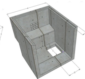
CORTE CÁMARA TIPO A (M.T-A) RED MEDIA TENSIÓN
