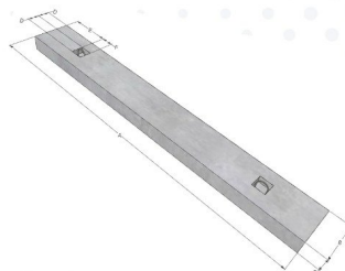
TAPA DE HORMIGÓN ARMADO (48,3 KG POR UNIDAD APROX.)
