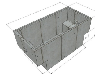
CÁMARA TIPO A (M.T-A) RED MEDIA TENSIÓN
