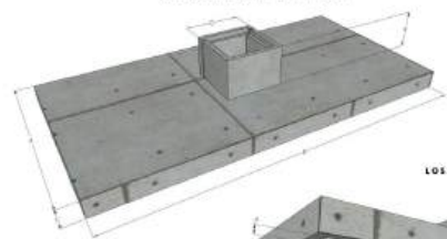
LOSA CÁMARA TIPO A - VISTA A
